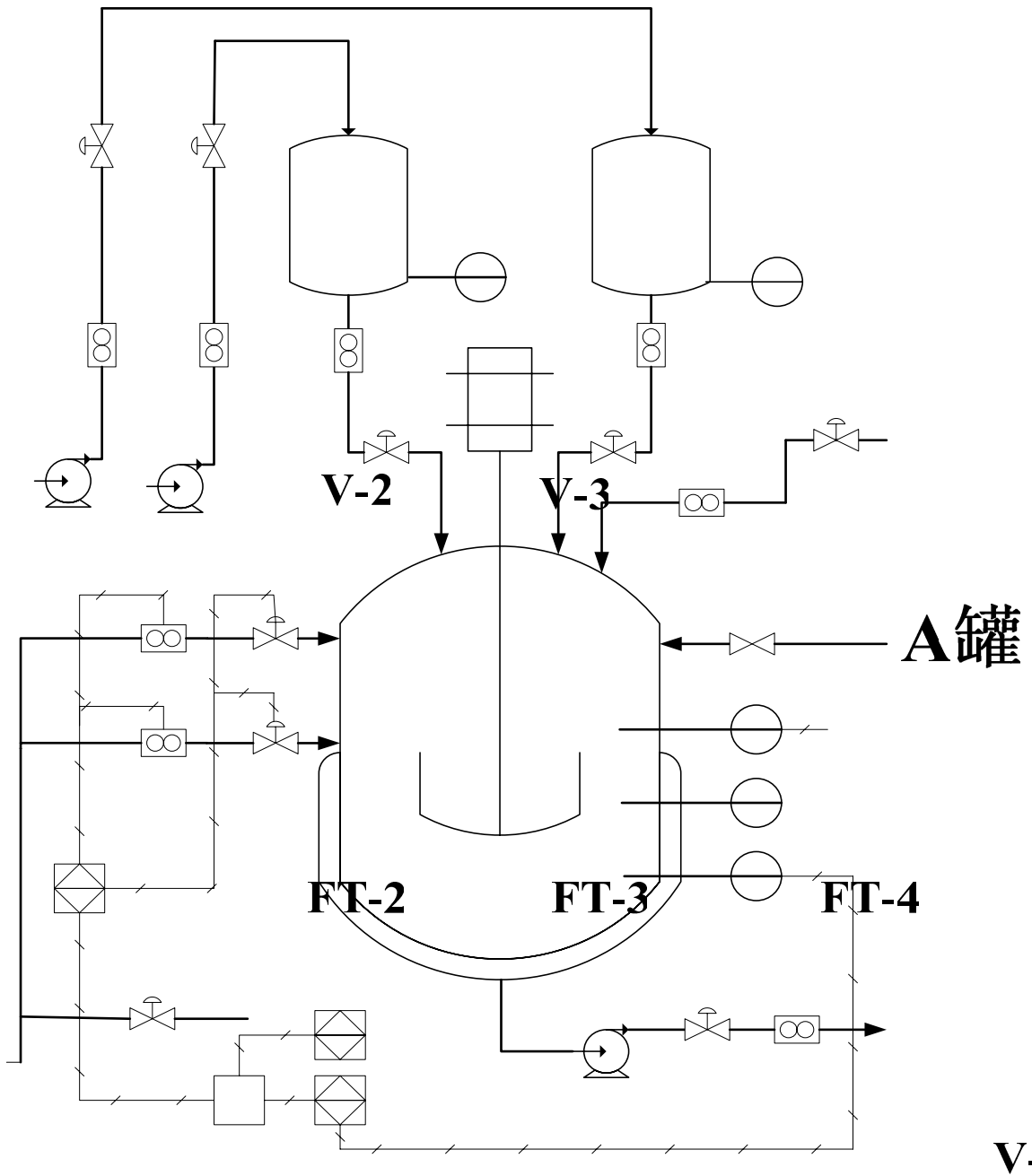
图 2.9 恒温控制 P&ID 图
